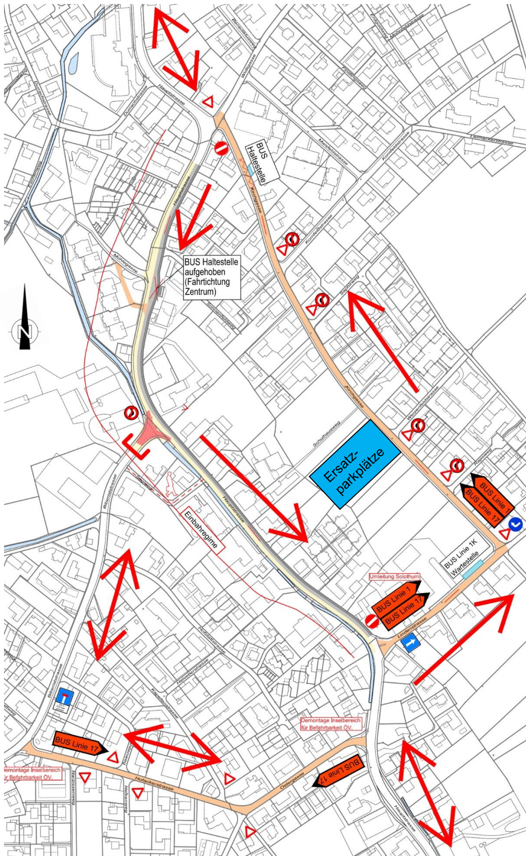
Abbildung 2 – Verkehrsführung Phase 2 (September 2024 - Februar 2025)
