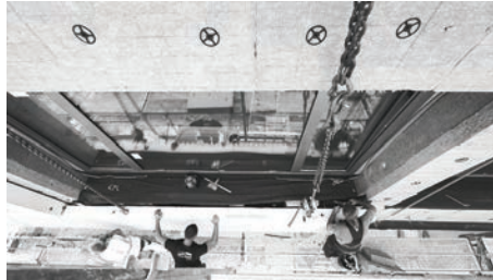
Schultrakt Ostfassade. Arbeiter beim Montieren der vorfabrizierten Betonelemente.
